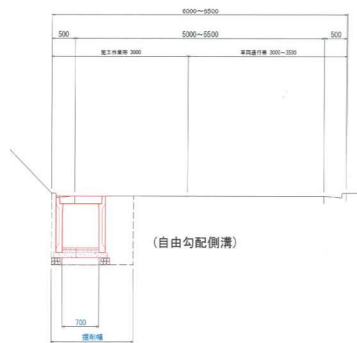
標準断面図
