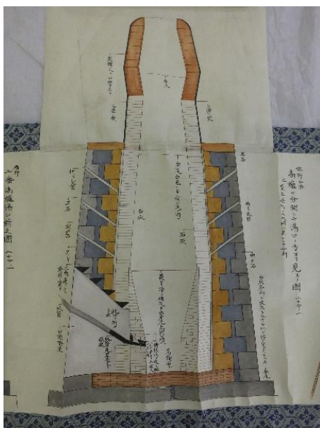
上：湯口前働の図
