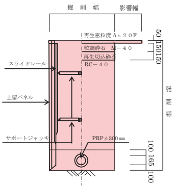
標準断面図
