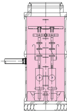
標準断面図
