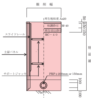
標準断面図
