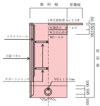
標準断面図
