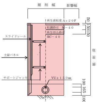
標準断面図
