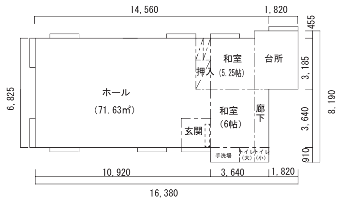
洞泉市営住宅自治会集会所 平面図 S=1/100
