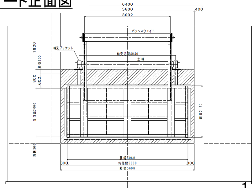
ゲート正面図
