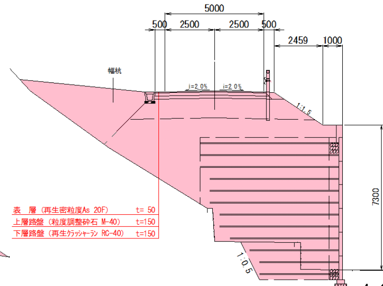
横断面図(補強土壁部)
