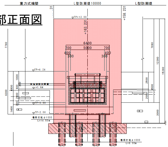
ゲート正面図
