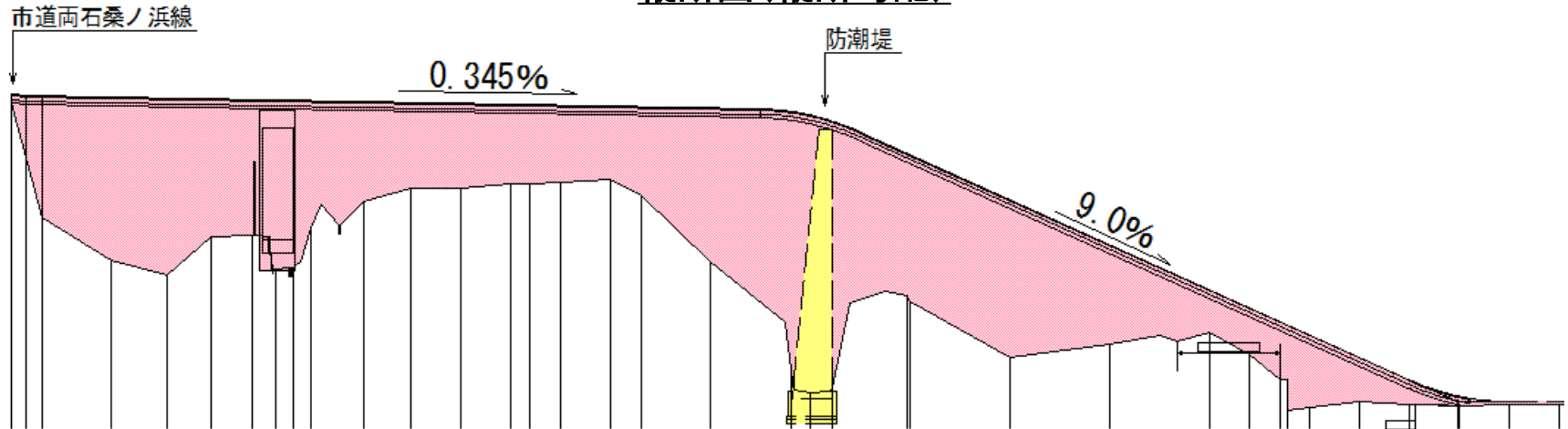
縦断面図(縦断勾配)
