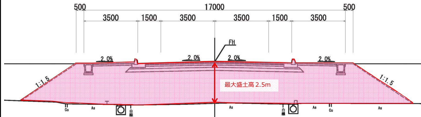
国道45号標準横断図
