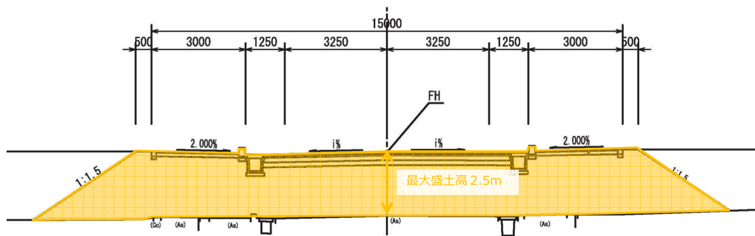
国道283号標準横断図
