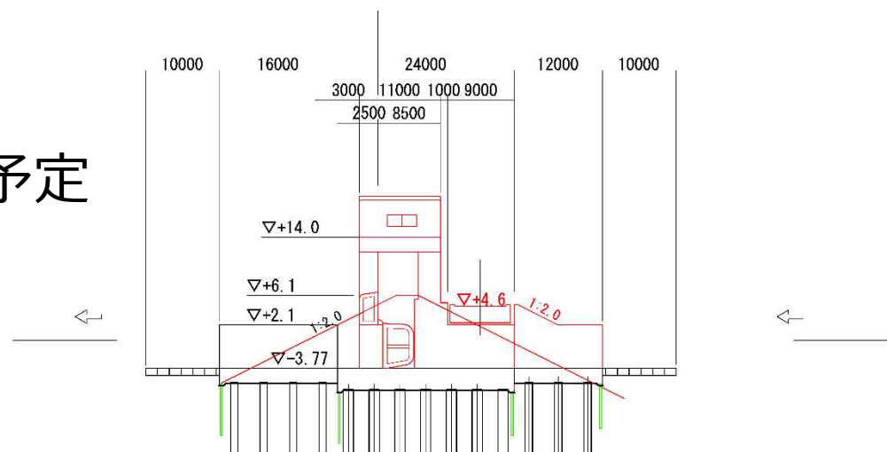
側面図
