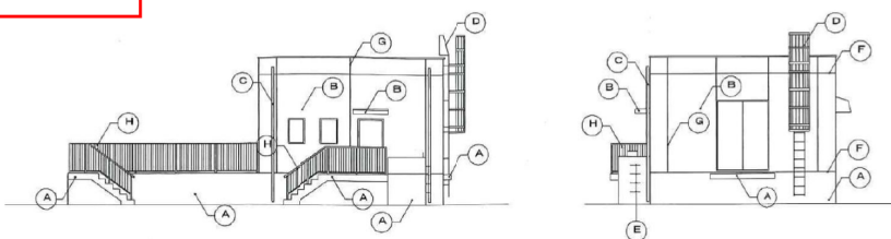
施設立面図
