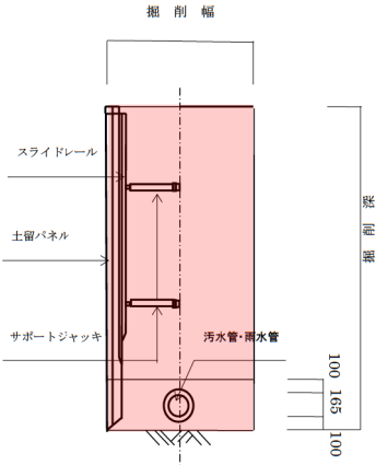
標準断面図
