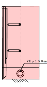
標準断面図
