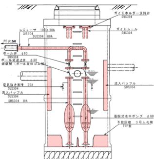
標準断面図
