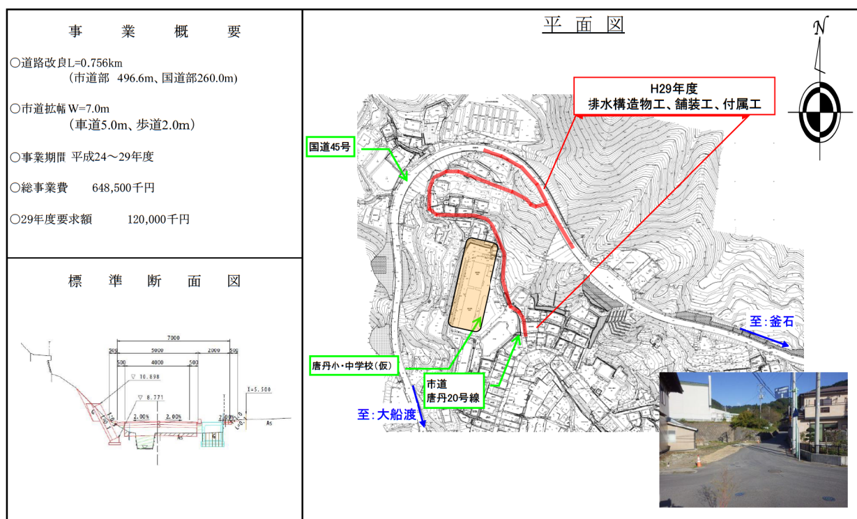
唐丹20号線道路改良工事 計画平面図
