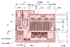
簡易処理高度化施設 平面図
