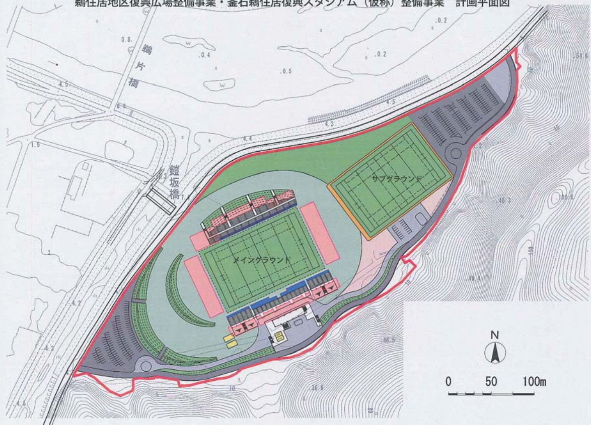
鶴住居地区復興広場整備事業・釜石鶴住居復興スタジアム（仮称）整備事業 計画平面図
