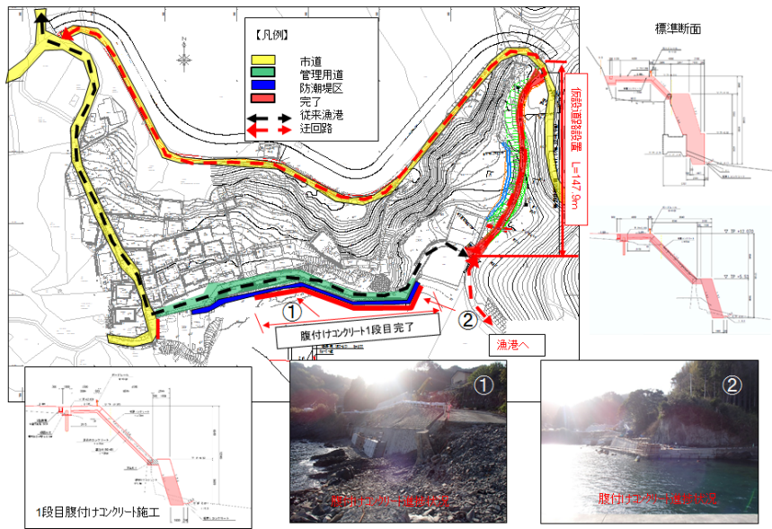
仮宿漁港防潮堤進捗状況 (H28.5月)
