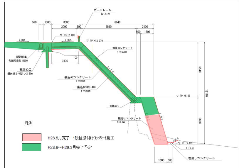
仮宿漁港防潮堤計画
