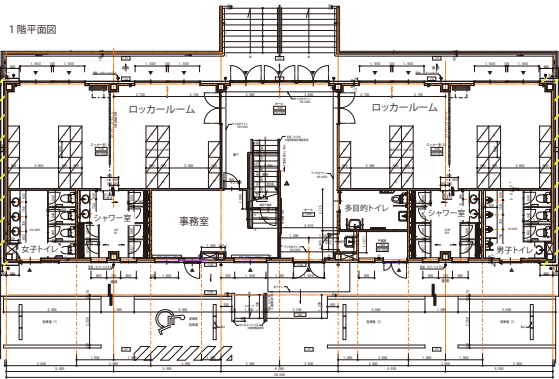
クラブハウス平面図
