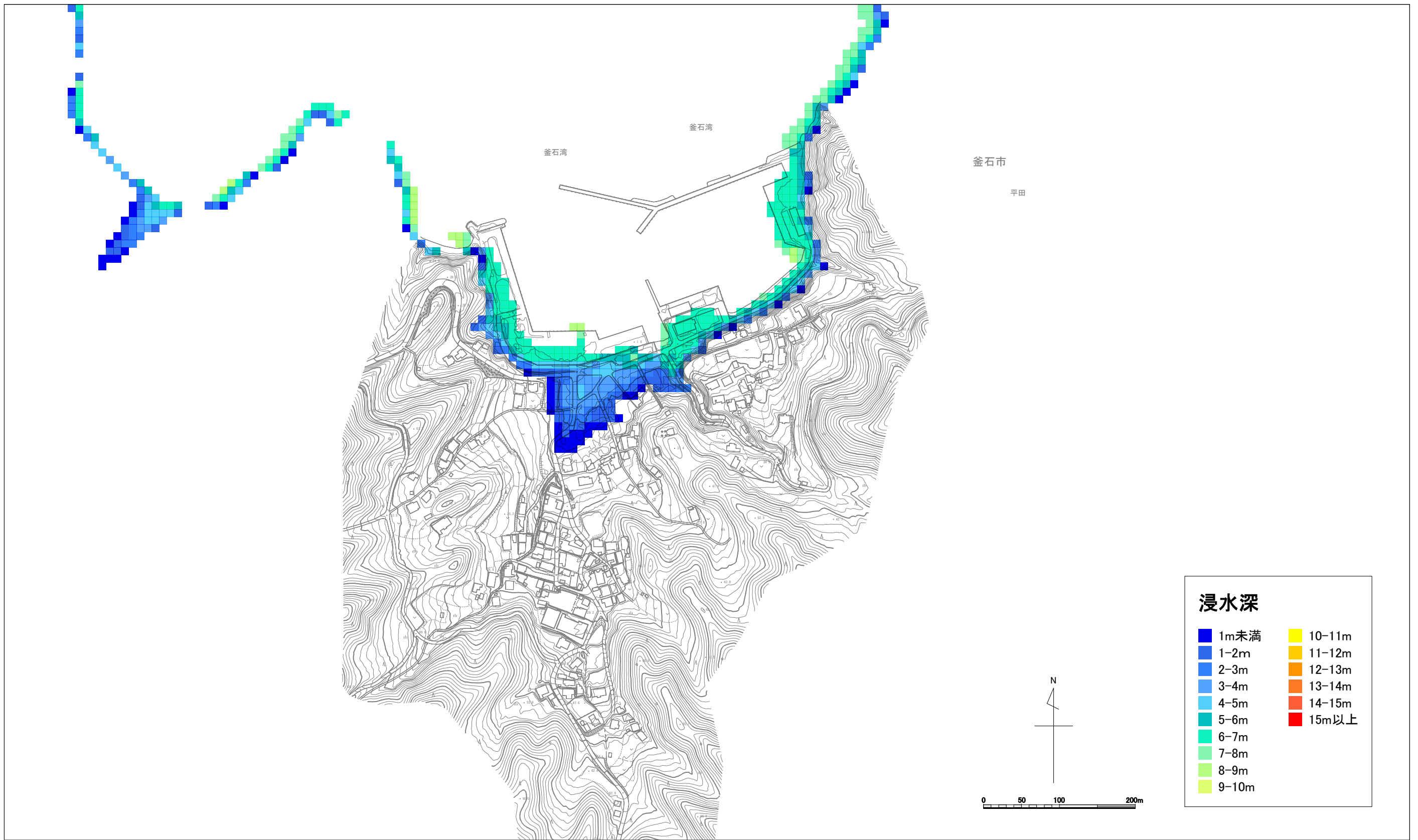
水門案：明治三陸津波を溢れさせない防潮堤高（T.P. 6.1m）におけるシミュレーション結果（尾崎白浜）
