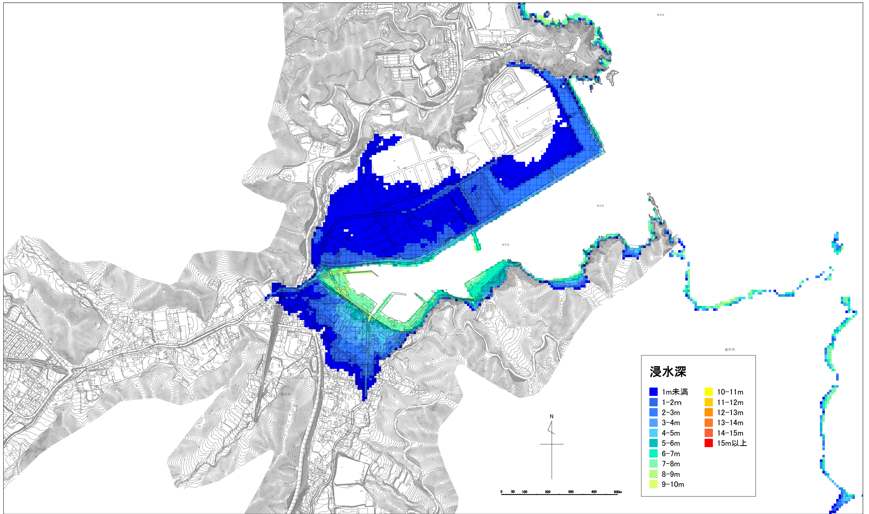
水門案：明治三陸津波を溢れさせない防潮堤高（T.P. 6.1m）におけるシミュレーション結果（平田）
