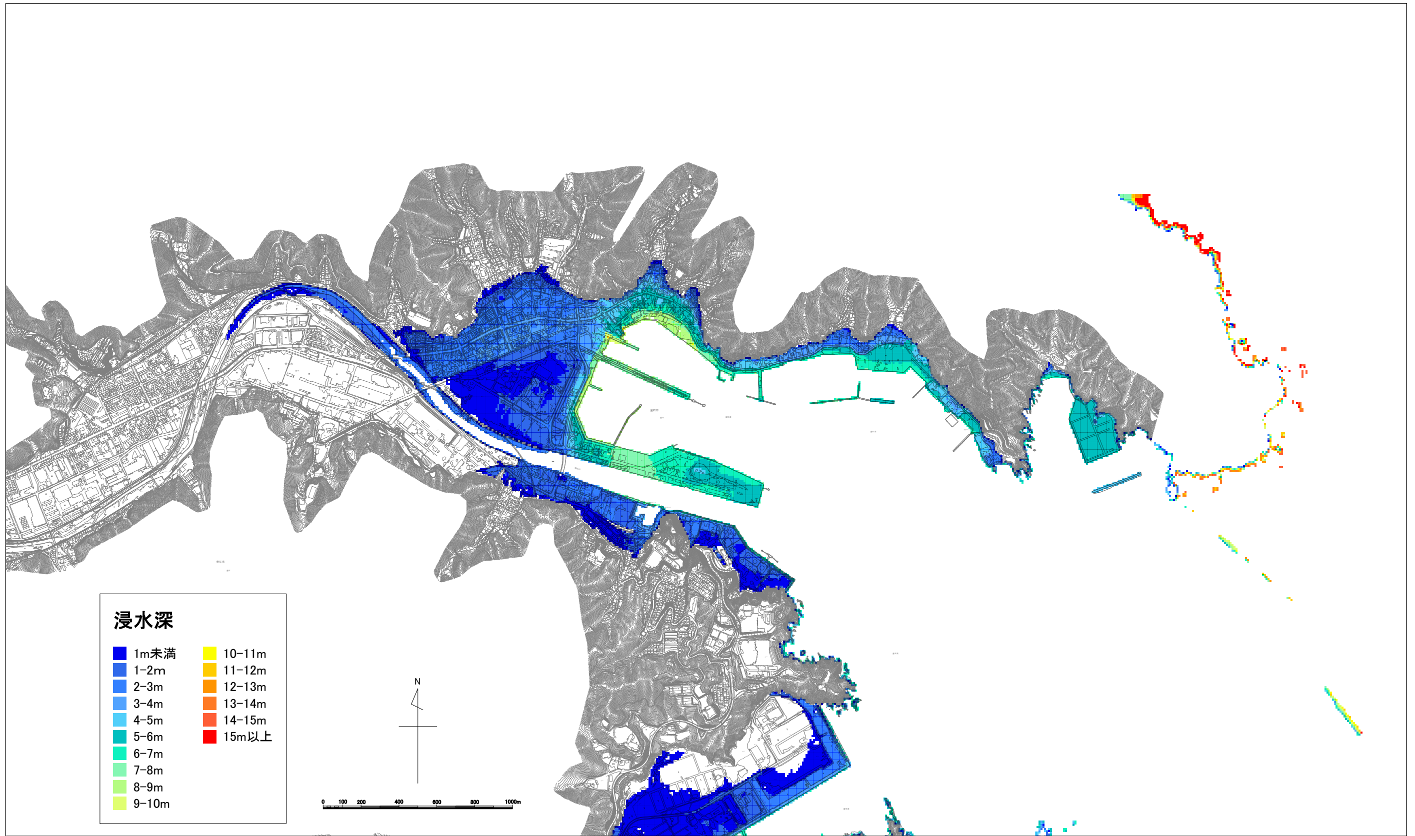
水門案：明治三陸津波を溢れさせない防潮堤高（T.P. 6.1m）におけるシミュレーション結果（東部地区）
