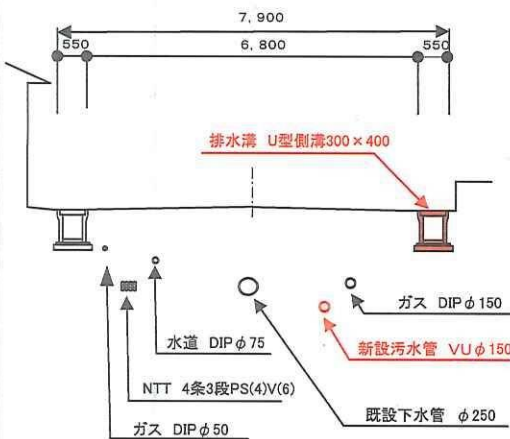
断面図
